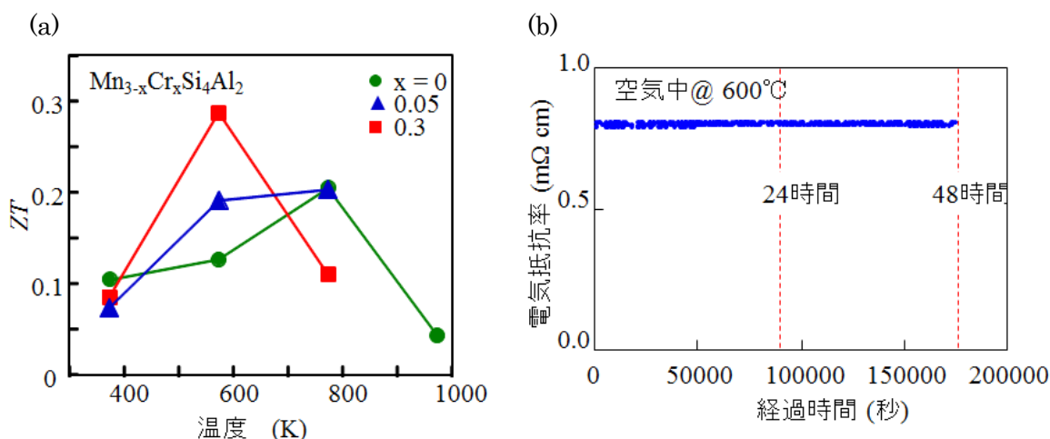
図 4 Mn_{3-x}Cr_xSi_4Al_2 の無次元性能指数 ZT の温度依存性(a)と Mn_3Si_4Al_2 焼結体の 600^\circ C 、空气中での電気抵抗率の経時変化(b)。
