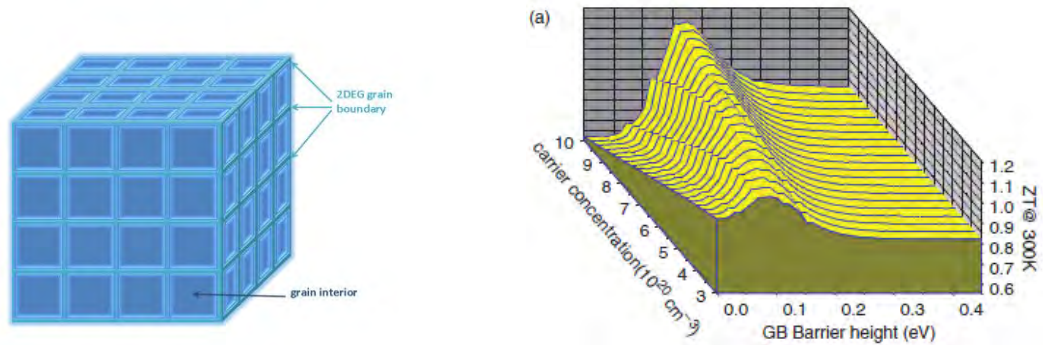
図 1 (a) 3D 超格子セラミックスの構造;粒子:La-SrTiO 3 、粒界:Nb-SrTiO 3 の2DEG 層; (b) 3D 超格子セラミックスの ZT と粒界バリア高さ及び粒内キャリア濃度の関係
