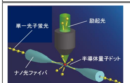
図 5. ナノ光ファイバ表面の半導体量子ドットからの単一光子蛍光の高効率結合
