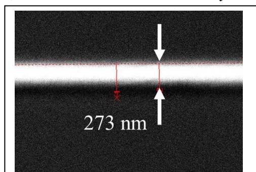
図 4. 光ファイバの一部を延伸して作成したナノ光ファイバの操作型電子顕微鏡像。延伸部直径は推定 273nm。
