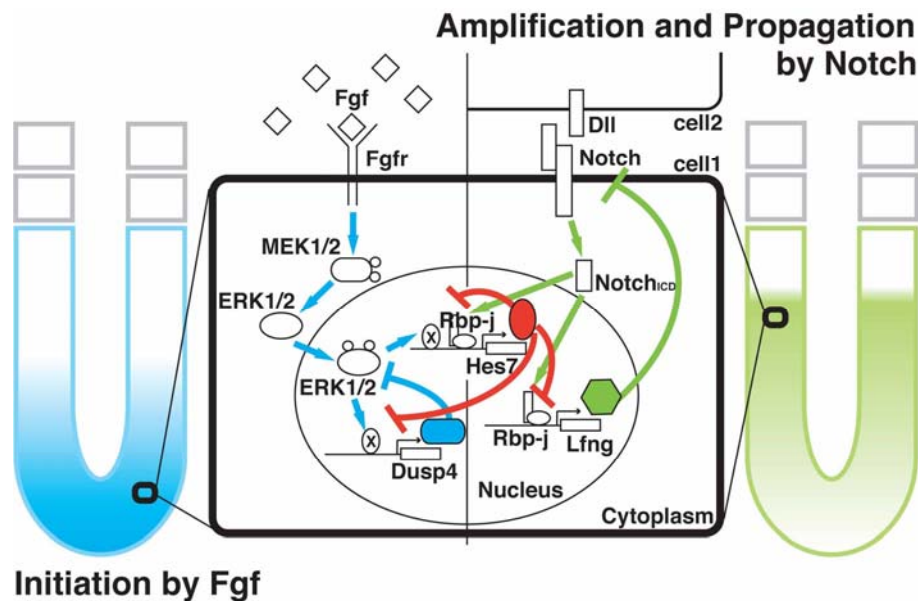
図5: 分節過程における Hes7 を中心としたオシレーションネットワーク
