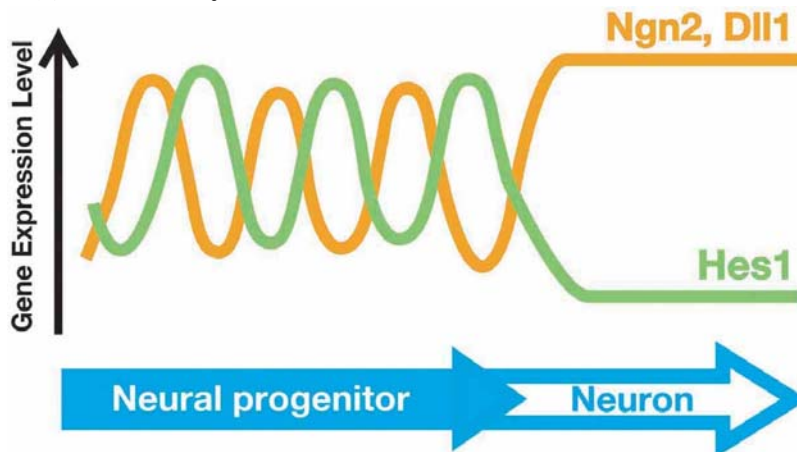
図9:神経幹細胞と分化途中のニューロンにおける Hes1,Ngn2,Dll1 の発現動態
