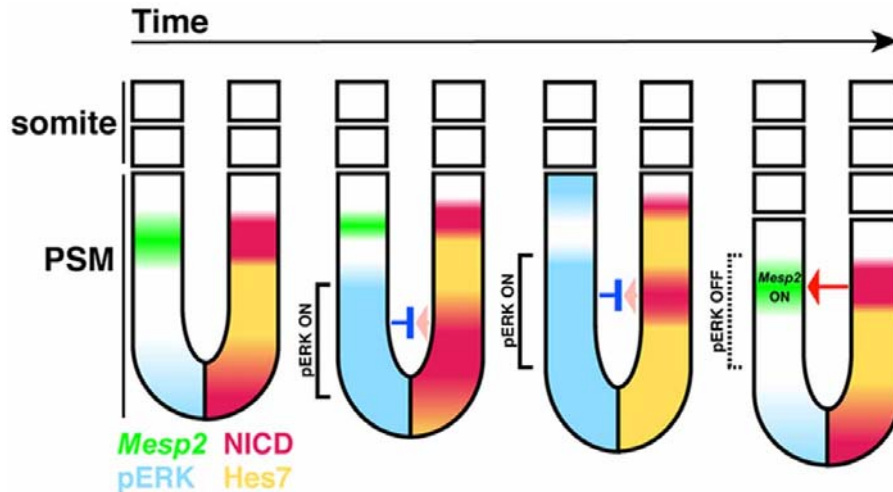
図6:分節過程での Hes7, Mesp2, NICD, pERK の発現動態。NICD と pERK の発現は未分節中胚葉の後端ではほぼ同じ位相で振動するが、前側では位相が逆転する。その結果、NICD は S1 領域全体に Mesp2 の発現を誘導する。
