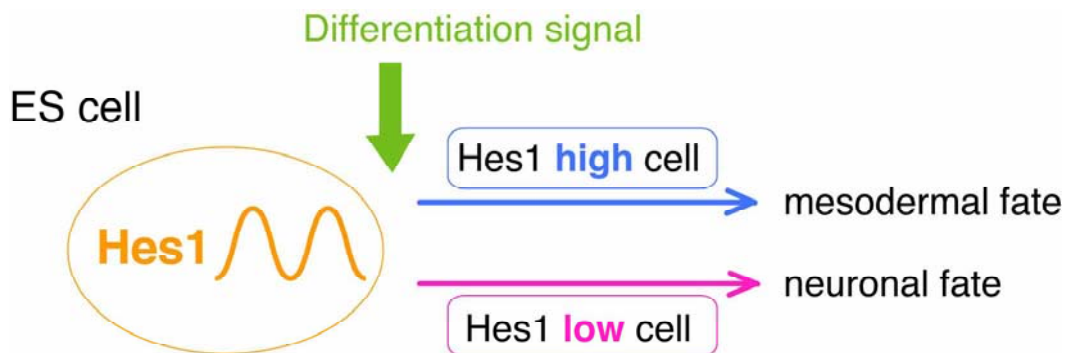
図12:ES 細胞の多様な分化応答に Hes1 オシレーションが寄与。ES 細胞では Hes1 の発現がオシ
