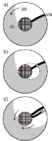
図16:心筋でピン止めされた回転らせん波の除去(模式図)
