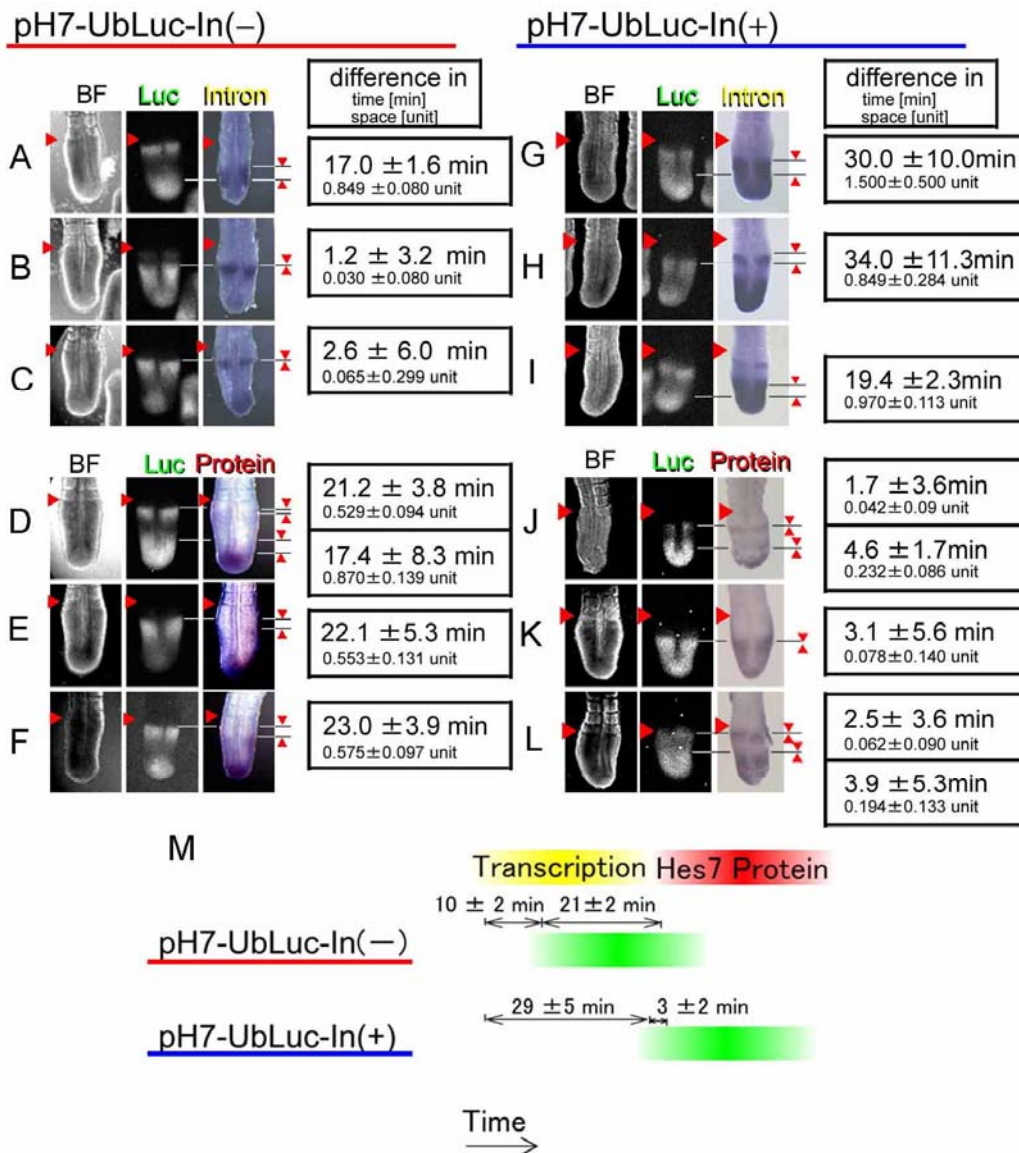
図2: Hes7 遺伝子のイントロンを含むレポーターと含まないレポーターの発現を内在性 Hes7 の発現と比較した。レポーターの発現は、イントロンの存在によって約19分遅れた。
