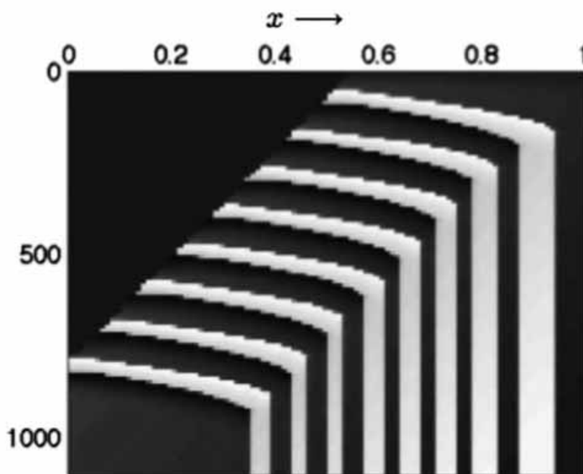
図14: 空間離散の数理モデルで得られた活性因子の空間分布の時間変化。
