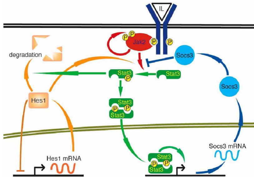
図8:線維芽細胞における Hes1 を中心としたオシレーションネットワーク
