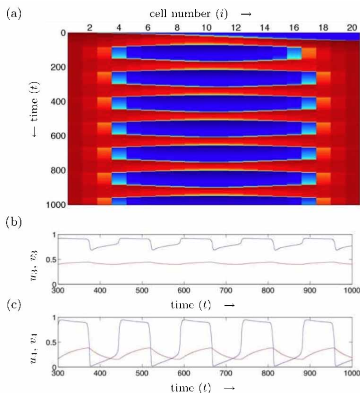
図13:細胞の振動状態と空間分布。色の違いは、細胞内部の反応回路が異なる回り方をしている事に対応する。それが分化に関わるものであれば、色に応じて分化していくであろう。
