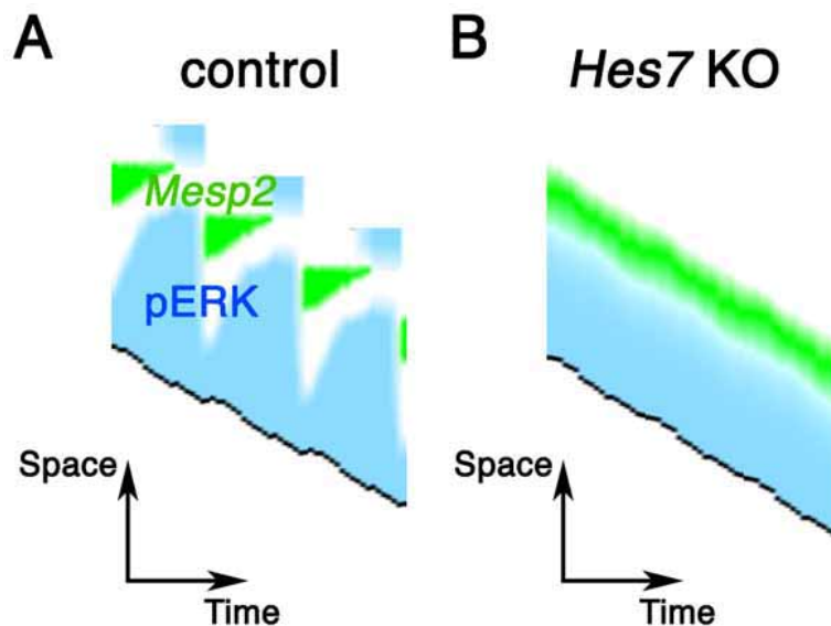
図7:pERK と Mesp2 の発現の時空間プロット。(A)正常では、pERK の発現が無くなると、NICD が Mesp2 の発現を誘導する。(B)一方、Hes7 遺伝子を欠損すると、NICD や pERK の発現振動が消失し、Mesp2 は S1 領域あたりを徐々に後側へ移動するように発現する。
