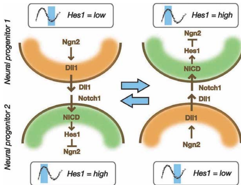
図10: 神経幹細胞における発現オシレーション。ある神経幹細胞の Delta1 の発現が高いと(左上)隣接する神経幹細胞の Notch シグナルを活性化し、その細胞の Hes1 の発現が増え、Ngn2 と Delta1 の発現が減る(左下)。しかし、オシレーションのために約1時間後には Hes1 の発現が減少して Ngn2 と Delta1 の発現が増加し(右下)、前者の神経幹細胞の Notch シグナルを活性化する(右上)。このように、神経幹細胞同士がお互いに Notch シグナルを活性化し、細胞集団全体の未分化性が維持される
