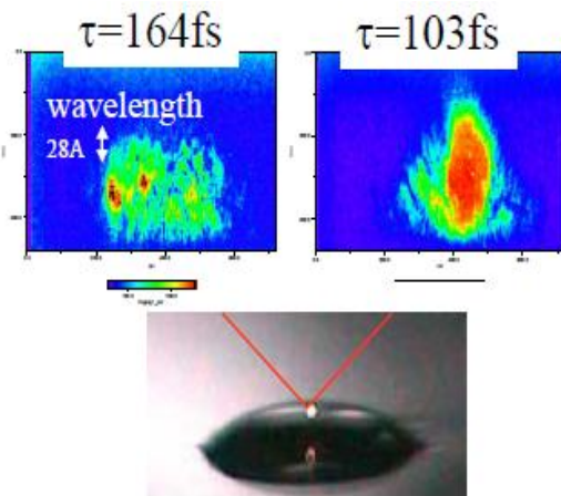
図 18. Warm dense matter 領域での金属-非金属転移を用いたフェムト秒光スイッチ
