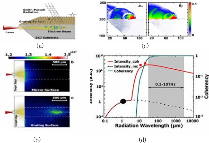
図14. (a)レーザー誘起電子ビームによるスミスパーセル放射の原理(b)グレーティング面と平面から放射(c)グレーティング構造を持った導体近辺での電子ビームガイドを誘起する自己生成電場と磁場(計算)(d) スミスパーセル放射の実験点とテラヘルツ領域の相対強度(計算)
