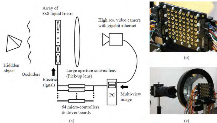
図 12 可変焦点レンズアレイによる 3 次元情報の取得
