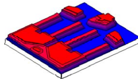
スライダ拡大図(上面がABS)
