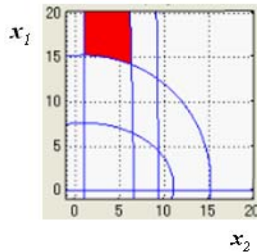
全ての仕様を満たす x_1 , x_2 の実行可能領域
