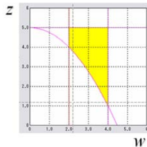
QE の計算例と実行可能解
