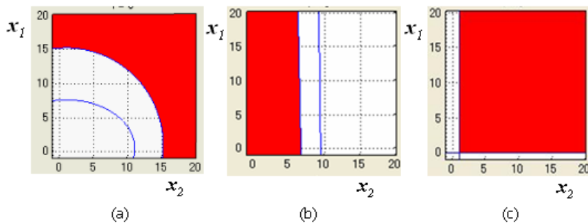
各仕様に対する x_1, x_2 の実行可能領域
