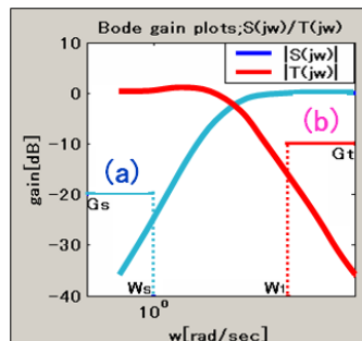
ボーデ線図における感度・相補感度の制約
