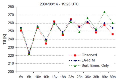
図 13 周波数別の輝度温度（観測値：赤、大気の影響を考慮しない陸面データ同化による陸面での計算輝度温度：緑、陸面での計算値を境界条件として大気の影響を考慮した大気上端での計算輝度温度：青）
