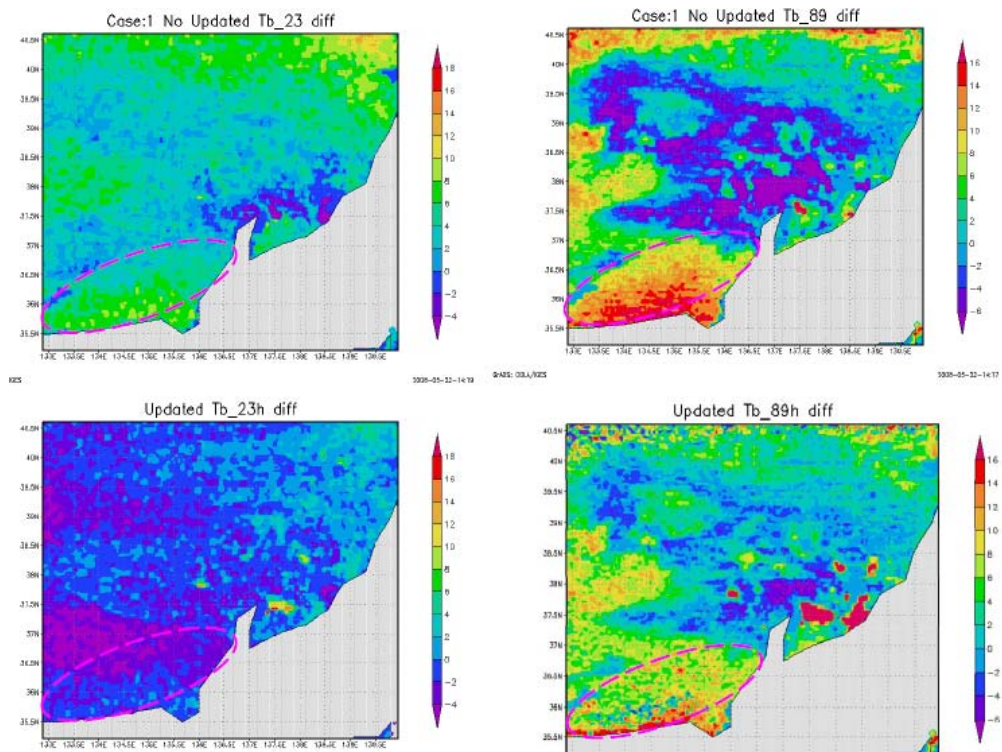
図 1 1 輝度温度の同化結果（上段：同化前、下段：同化後、左：23GHz、右：89GHz、ピンク点線で囲まれた領域の輝度温度の誤差が、同化後に著しく減じている。）
