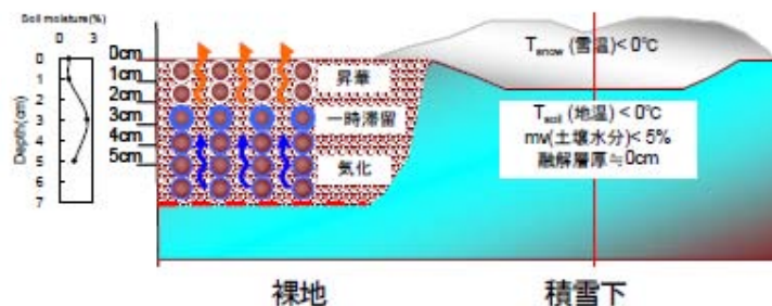
図26 チベット高原での積雪と裸地における凍土融解層の発達状況の違い
