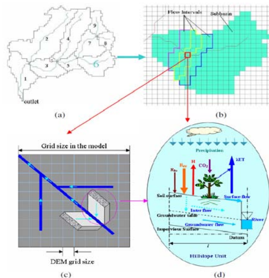
図 15 グリッド型 GBHM の構成：(a) 流域をサブ流域に分割、(b) 複数の Flow Interval からなるサブ流域、(c) Flow Interval を構成するグリッド (DEM グリッドにより斜面、河道が特徴づけられる)、(d) 各グリッド斜面に適用される陸面スキーム
