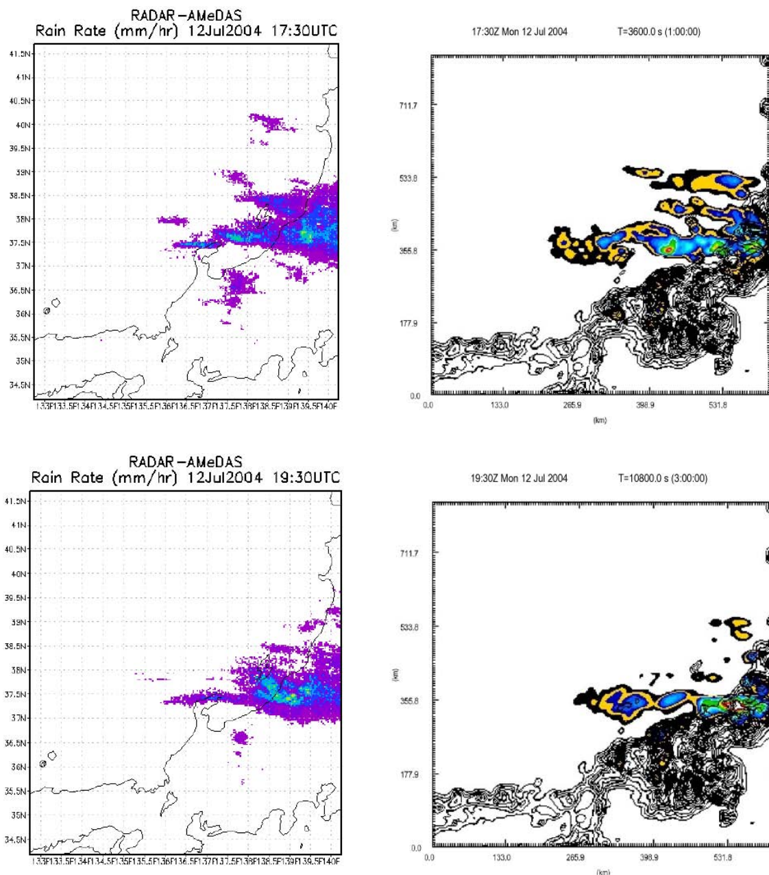
図 12 雲微物理同化システムを組み込んだ物理的ダウンスケーリングによる豪雨予測（上段：1時間先、下段：3時間先のレーダ・アメダスによる降雨分布観測結果（左）、予測結果（右））
