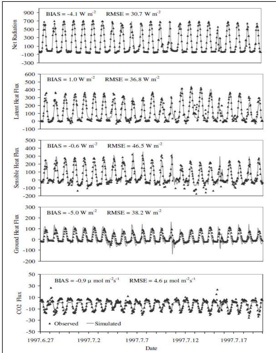
図 20 Little Washita 流域内のフラックス観測サイトで観測された各フラックス (▲、上から正味放射、潜熱、顕熱、地中熱流、二酸化炭素) と WEB-DHM の計算値 (実線)
