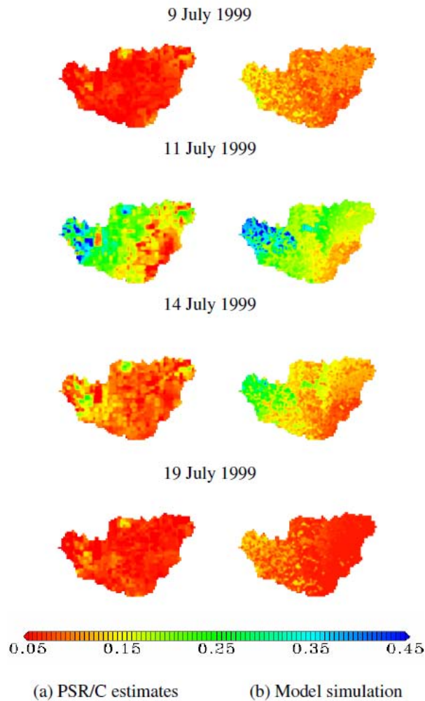
図 22 1999 年 SGP99 において航空機搭載マイクロ波放射計 (PSR/C) で観測された土壌水分(体積含水率%) 分布 (左) と WEB-DHM の算定結果 (右)
