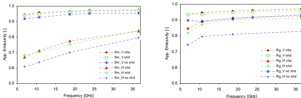
図5 Shadowing 効果を含んだ AIEM と稠密媒体の放射伝達モデル(DMRT)による砂層の放射伝達モデルの周波数ごとの見かけの放射率の検証結果 (左: なめらかな面、右: 人工粗度を付加した面)。観測値 (赤) に対して、Shadowing 効果を含まないもの (青) は特に水平偏波 (+) で観測値から離れているのに対して、Shadowing 効果を含む (緑) 結果は水平 (○)、垂直 (□) 偏波いずれも全周波数にわたって観測値に近い。
