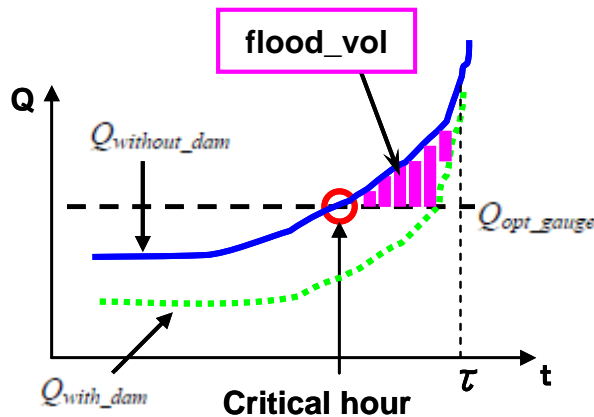
図 23 洪水調節と水利用を最適化するためのスキーム
