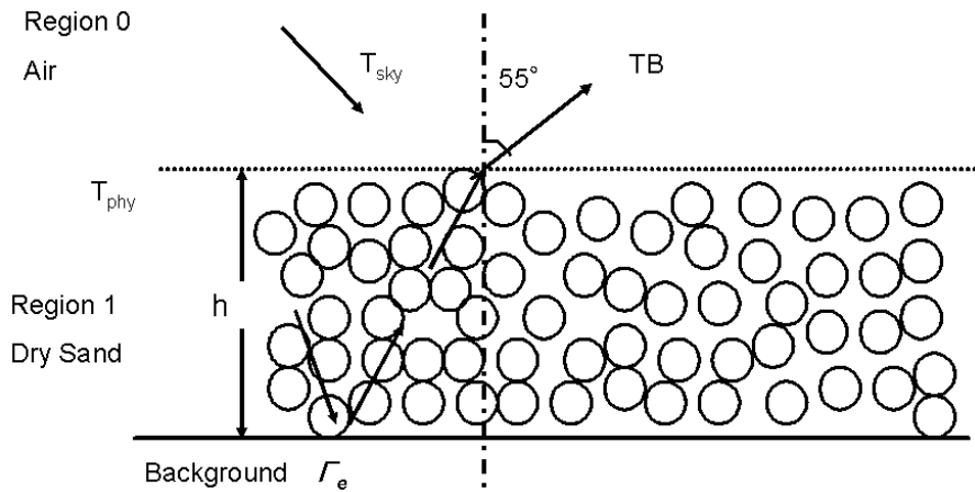
図2 放射伝達モデルの幾何的な構成
