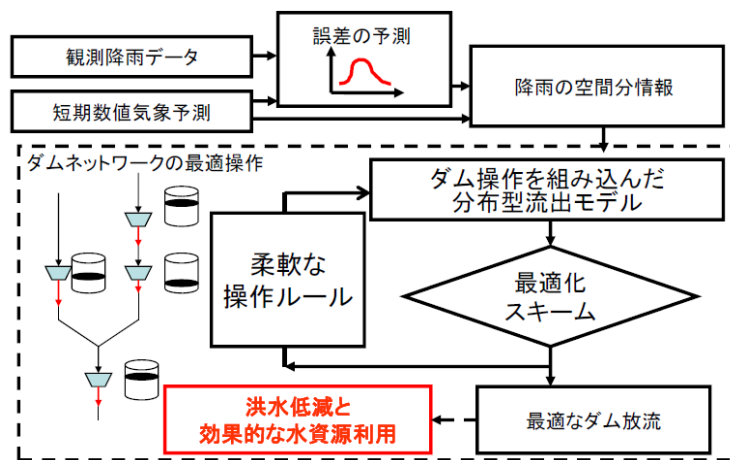
図 24 気象予測値と分布型流出モデルを組み合わせたダム最適操作システムの概要
