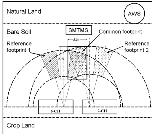
図1 2台のマイクロ波放射計による地上観測実験 (左：観測風景，右：共通のターゲット領域)
