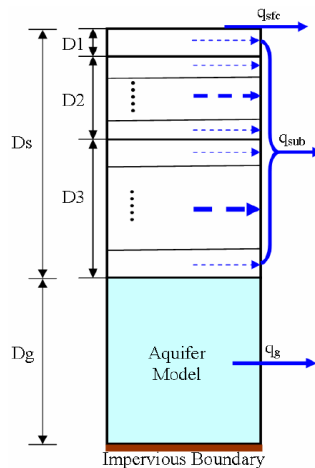
図 17 陸面スキーム (SiB2) のサブレイヤ化と地下水層の追加および側方流出成分
