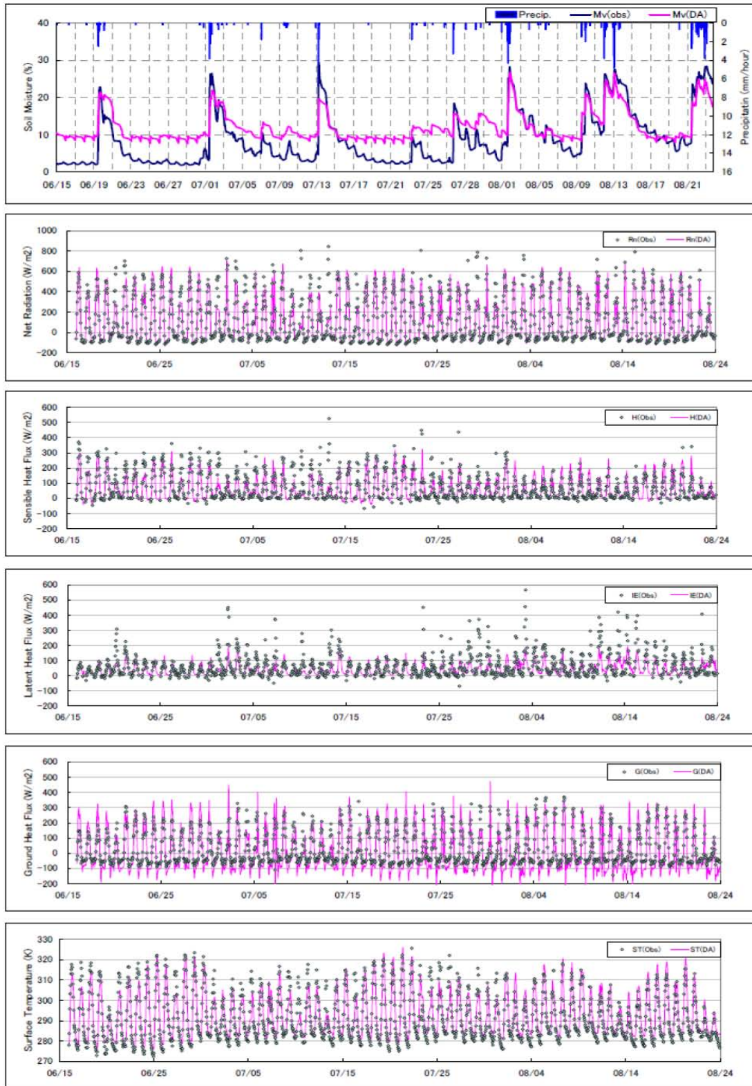
図9 2007年6月16日～8月23日における、CEOPチベットGaize観測所への陸面データ同化の適用結果。(上段より、降水量と土壌水分、正味の放射収支、顕熱フラックス、潜熱フラックス、地中熱流量、地表面温度。フラックスはボーエン比法により算定。ピンク線がデータ同化結果、青線もしくは青点が観測値。)
