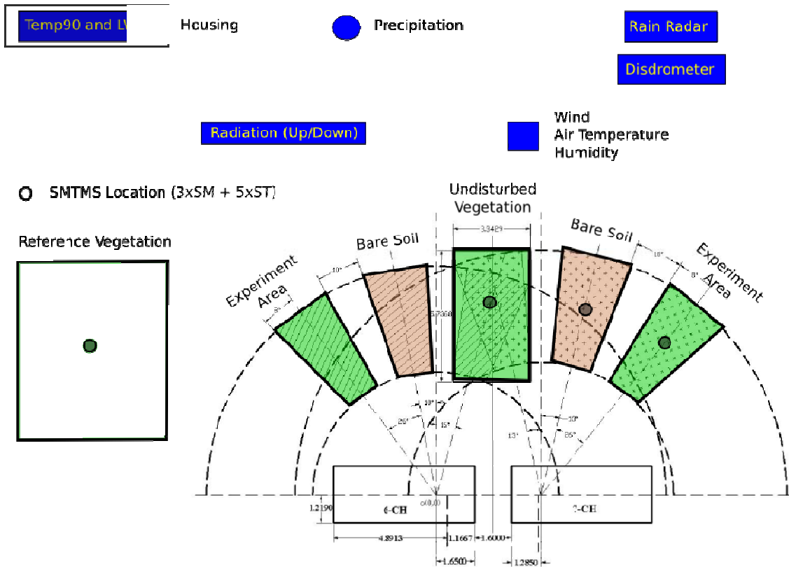
図7 東大農場における2台のマイクロ波放射計を用いた植生観測実験
