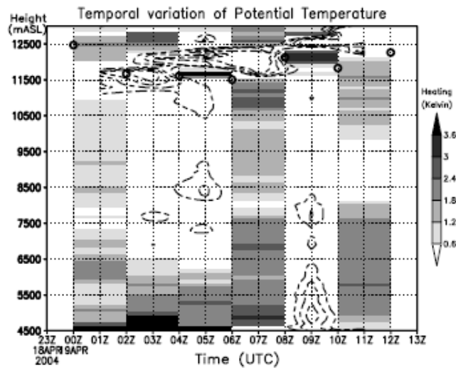
図 27 ラジオゾンデ観測結果を用いた各 2 時間毎の大気昇温量。破線は負の値を示し、等値線間隔は 0.6K。白丸はゾンデ観測より算定された対流圏界面 (2004 年 4 月 19 日)
