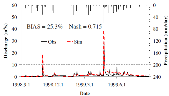
図 21 Little Washita 流域における WEB-DHM の検証結果
