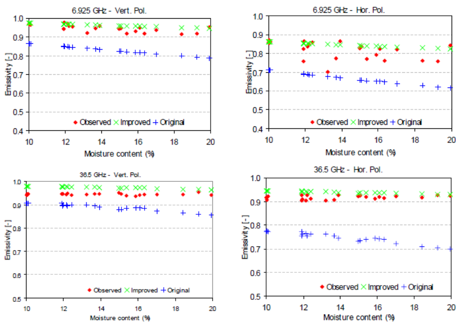
図6 CEOP モンゴルリファレンスサイトでの土壌マイクロ波放射伝達モデルの検証結果。6.9GHz (上段)、36.5GHz (下段) の垂直 (左)、水平 (右) 偏波において、体積含水率 10-20% まで観測放射率 (●) に対して、Shadowing を含まないもの (+) は水平偏波で低めに推定されるが、Shadowing を含めた結果 (×) は観測値とよく一致している。
