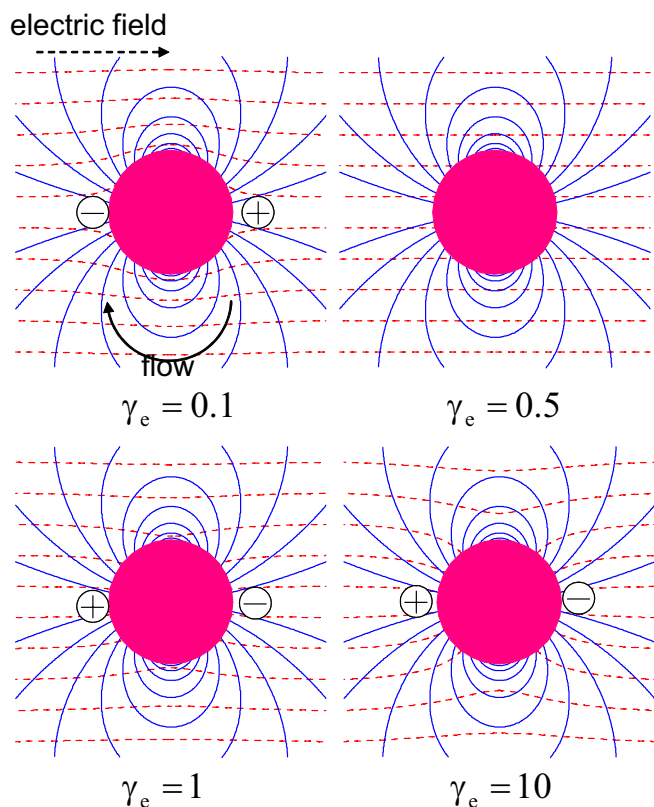
図 10: 電気泳動時における粒子の周りの電場。赤い破線が電場、青い実線が流れ場を表す。
