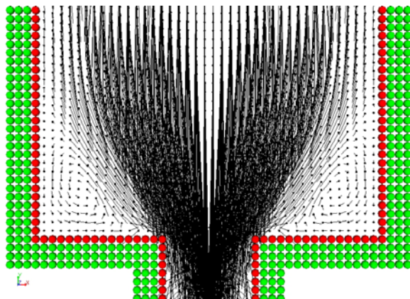
図 13: 狭窄流路中での contraction flow
