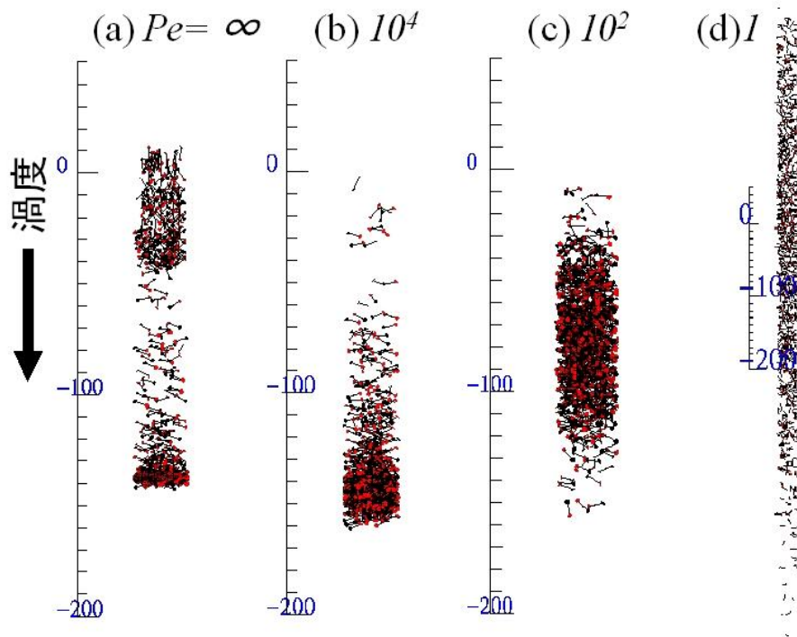
図2:単純せん断流におけるカイラリティを持つ粒子の運動。Pe はペクレ数と呼ばれる無次元数で、せん断流の強さと熱運動の効果の比を表す。(a),(b),(c),(d) の順に熱運動の効果が強い
