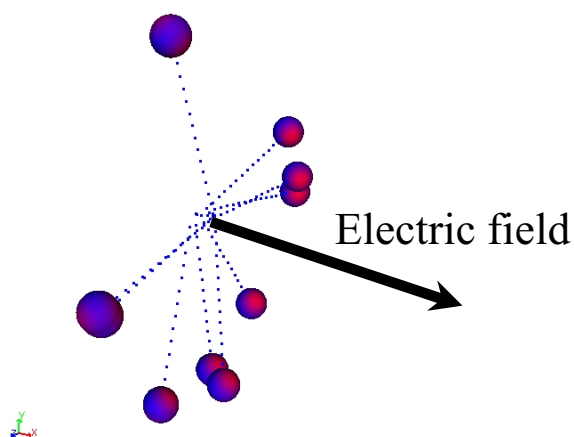
図7:非一様に荷電した粒子の電場の中の運動。粒子は電場と垂直方向に運動している。
