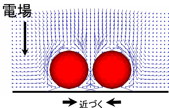
図8：電極付近で凝集する荷電粒子
