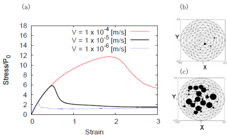
図 28 3D ブロックモデルにおける結果。(a) 3つの異なる引離し速度における応力-歪み曲線。 V = 1 \times 10^{-5} m/s での (b) \epsilon = 0.48 , (c) \epsilon = 1.5 におけるキャビティ生成の様子。
