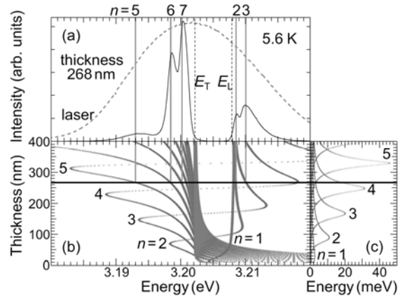
図 2.1 TG スペクトルと固有モード
