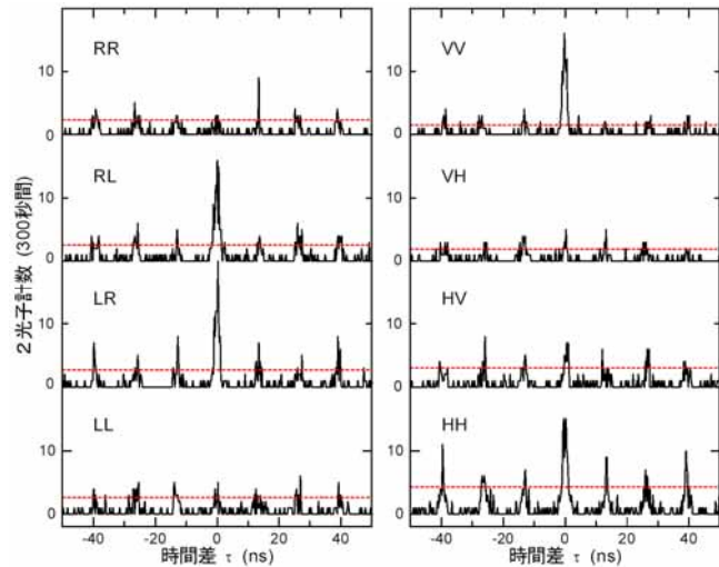
図3.1 発生した光子対の偏光相関の測定例。横軸は2光子の時間差、縦軸は2光子を検出した計数である。図中のRL、VH等の記号は、初めの文字が一方の光子の偏光方向、2番目の文字が他方の光子の偏光方向であり、R(L)が右(左)回り円偏光、V(H)が垂直(水平)方向の直線偏光を表す。互いに逆回りの円偏光(LRとRL)または互いに平行な直線偏光(HHとVV)の組み合わせのときのみ、 \tau=0 における同時検出信号が強く現れる。時間差 \tau が0以外の時に観測されるピークは、異なる励起光パルス(13 ns 間隔)によって生じた別々の励起子分子から放出された光子間の偶然の2光子計数であり、点線はその平均値である。
