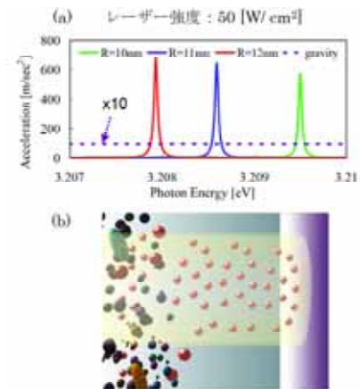
図4.4：(a)半径の異なる単一の球状半導体量子ドット (CuCl) に共鳴光が及ぼす輻射力による加速度の周波数依存性の計算結果。(b) 左からの伝播光による散乱力・吸収力で選別されたナノ微粒子を右端の基板上に輸送(概念図)。
