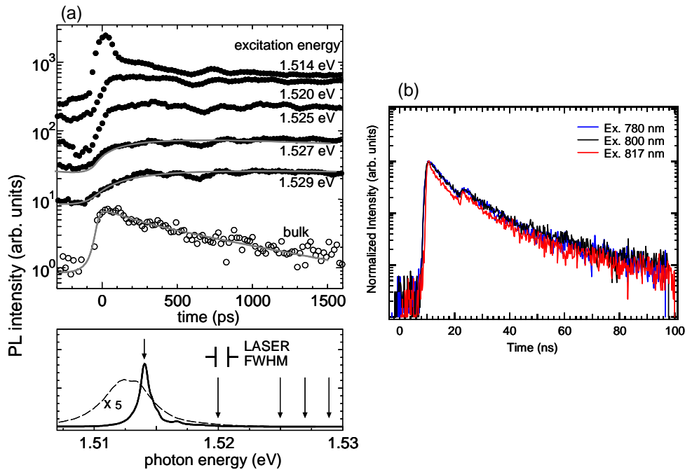
図1.5 (a)時間分解PL強度とPLスペクトル (b)繰り返し4MHz による時間分解PL
