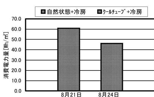
図1 冷房消費電力量の日積算値
