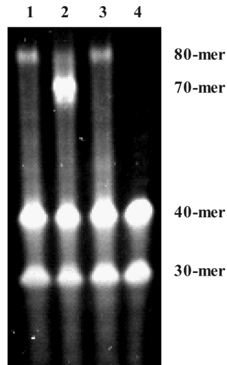
図1 . Tk-Lig のDNA ligase活性。 80 bの1本鎖DNAを鋳型とした際の30 b、40 bの1本鎖DNAの結合を指標に活性を測定している。 Lane 1は反応前、lane 2は反応後、lane 3はATP無添加、lane 4は鋳型無添加。
