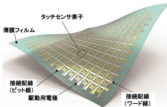
図2 柔らかいタッチセンサーシステムの構成
