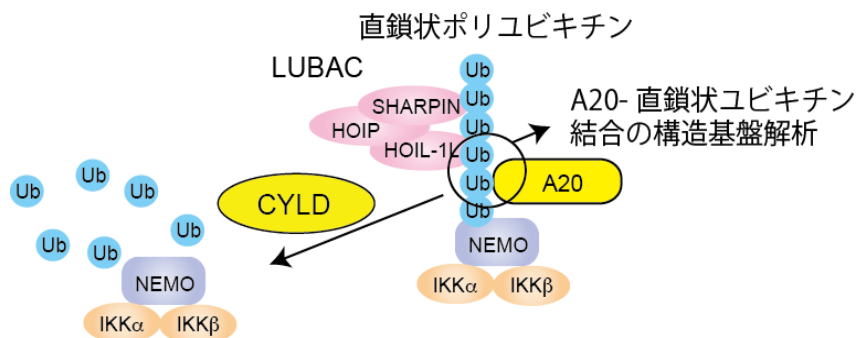
図 5. CYLD と A20 は異なる分子メカニズムで直鎖状ユビキチン化を介する NF-κB 活性制御を司る
