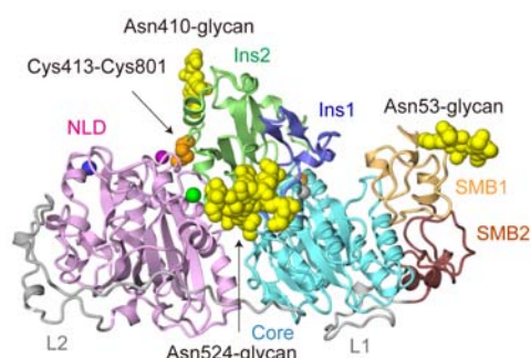
図1. ENPP2の結晶構造
