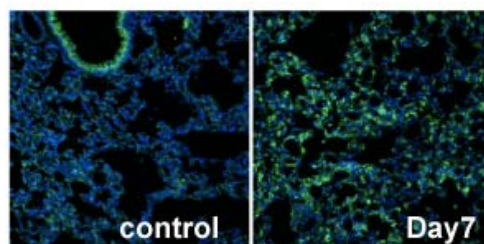
図 3. 肺線維症モデルにおける ENPP2 の発現上昇
